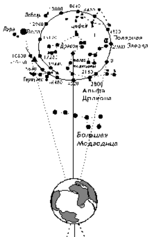
Смещение Полюса Мира в ходе Прецессии (Около 2000 года Северный Полюс вблизи звезды \alpha Малой Медведицы)
