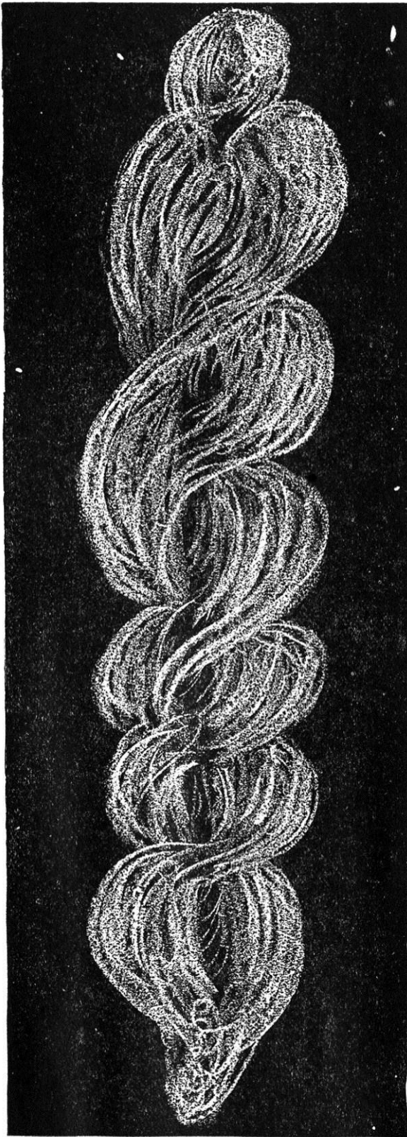
Рисунок 3. Первичный Вихрь. Сила, создающая планеты. Первый век вихря и начало существования кометы. Смерч в эфирийных небесах. Типичный диаметр — от полумиллиона до четырёх миллионов миль. Типичная длина — от 10 миллионов до 300 миллионов миль. [800 тыс. — 6,5 млн. и 16 млн. — 483 млн. км соответственно.]
