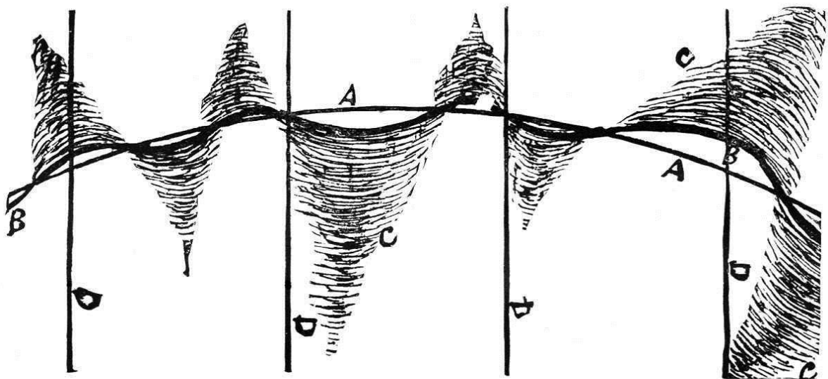
Рисунок 15. Отклонение Линии Солнечного Вихря. A, A — ход движения [справа налево (см. направление для круга 1 в Книге Знания, глава 4, рис. 1)] вихря Тау'сэн или семьи солнца Великого Змея. B, B — отклонение (вихря) от прямой линии. C, C — вихри с иными признаками миров. D, D — дэны, т.е. от D до D — три тысячи лет. Промежуток на кривой B рядом с центром рисунка показывает место, где сейчас находится Змей [≈32 г. к.].
