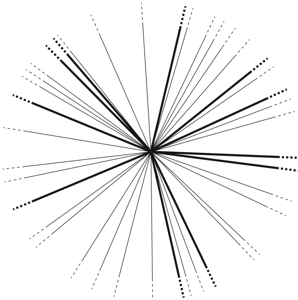
Рис. 4. Радиальная модель Вселенной
