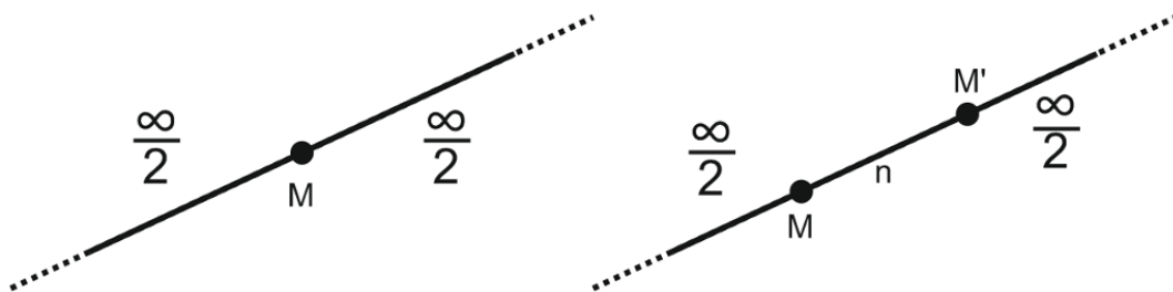
Рис. 3. Деление бесконечной прямой
